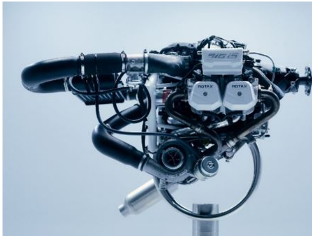
Il nuovo sistema di propulsione aeronautica Rotax 916iS/c
